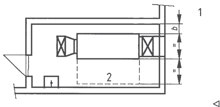
Figura 6.6.1. – Dispunerea instalațiilor de tratare a aerului (vedere în plan)
