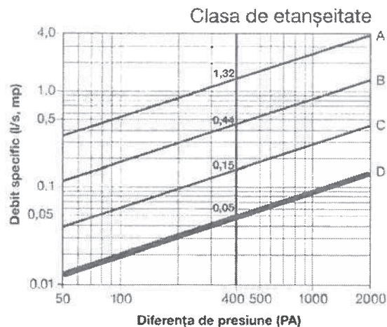
Fig. 6.2.1. Pierderile de aer maxime admise pentru cele 4 clase de etanșeitate
