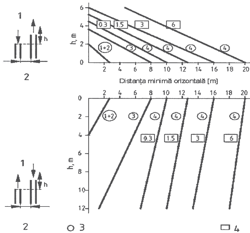
Figura 6.6.2. – Distanțe minime între gura de evacuare și cea de introducere a aerului Legendă: 1 Distanță verticală – Gură de evacuare deasupra prizei de introducere (partea superioară a graficului); Distanță verticală – Gură de evacuare sub gura de introducere (partea inferioară a graficului); 2- Distanță dintre prize; 3 - Categoria EHA ; 4 - Debit de aer în priză în m^3/s
